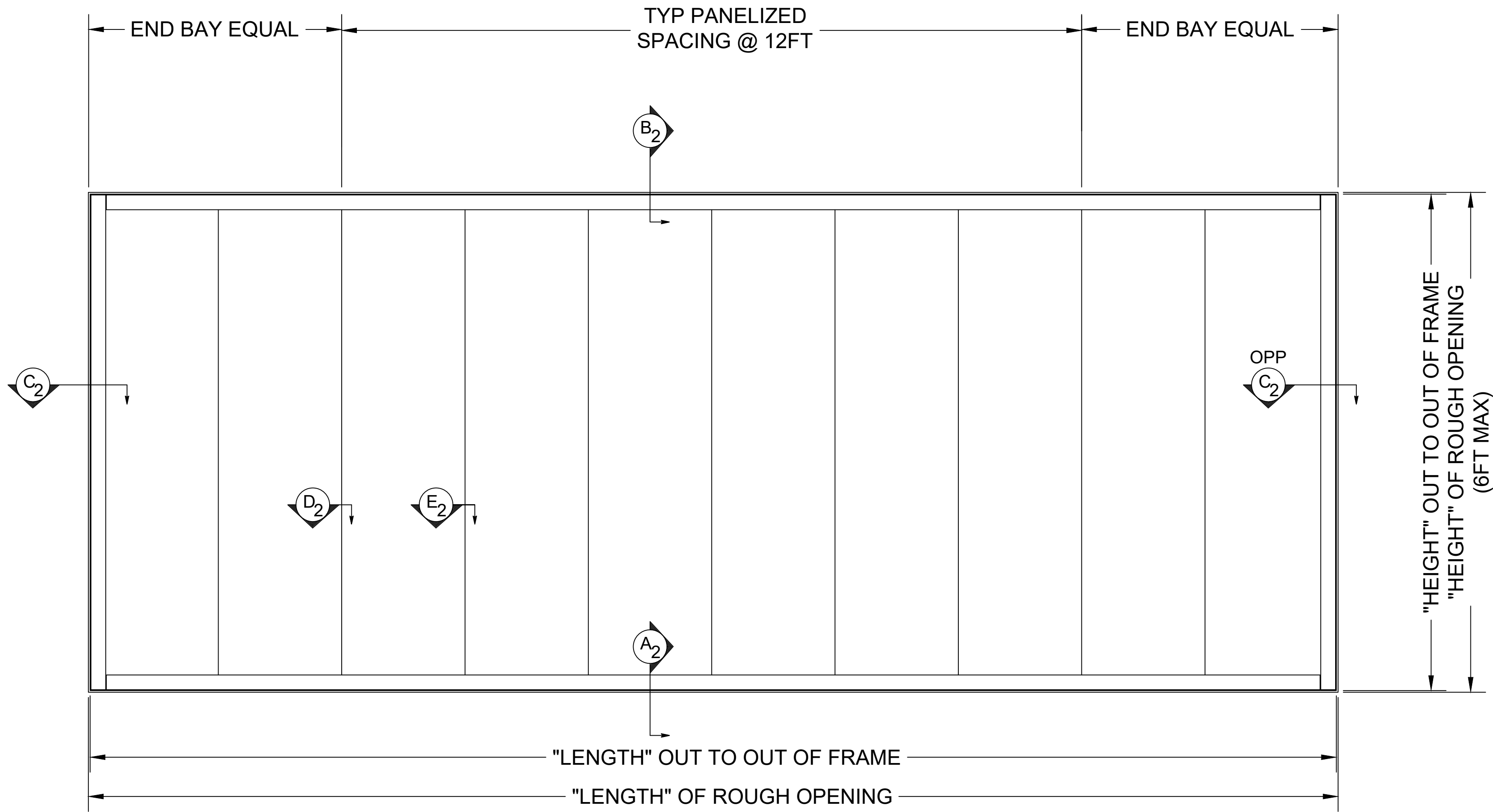
ELEVATION
