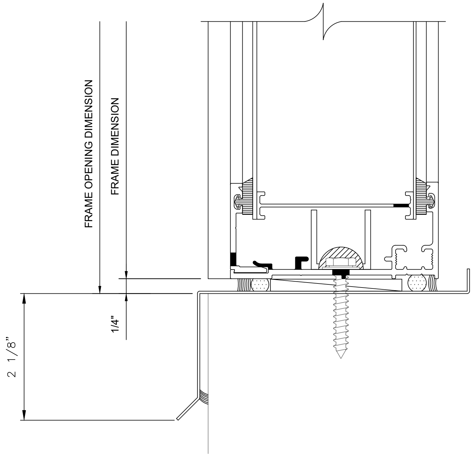
2 2 - - SILL DETAIL SCALE: FULL
