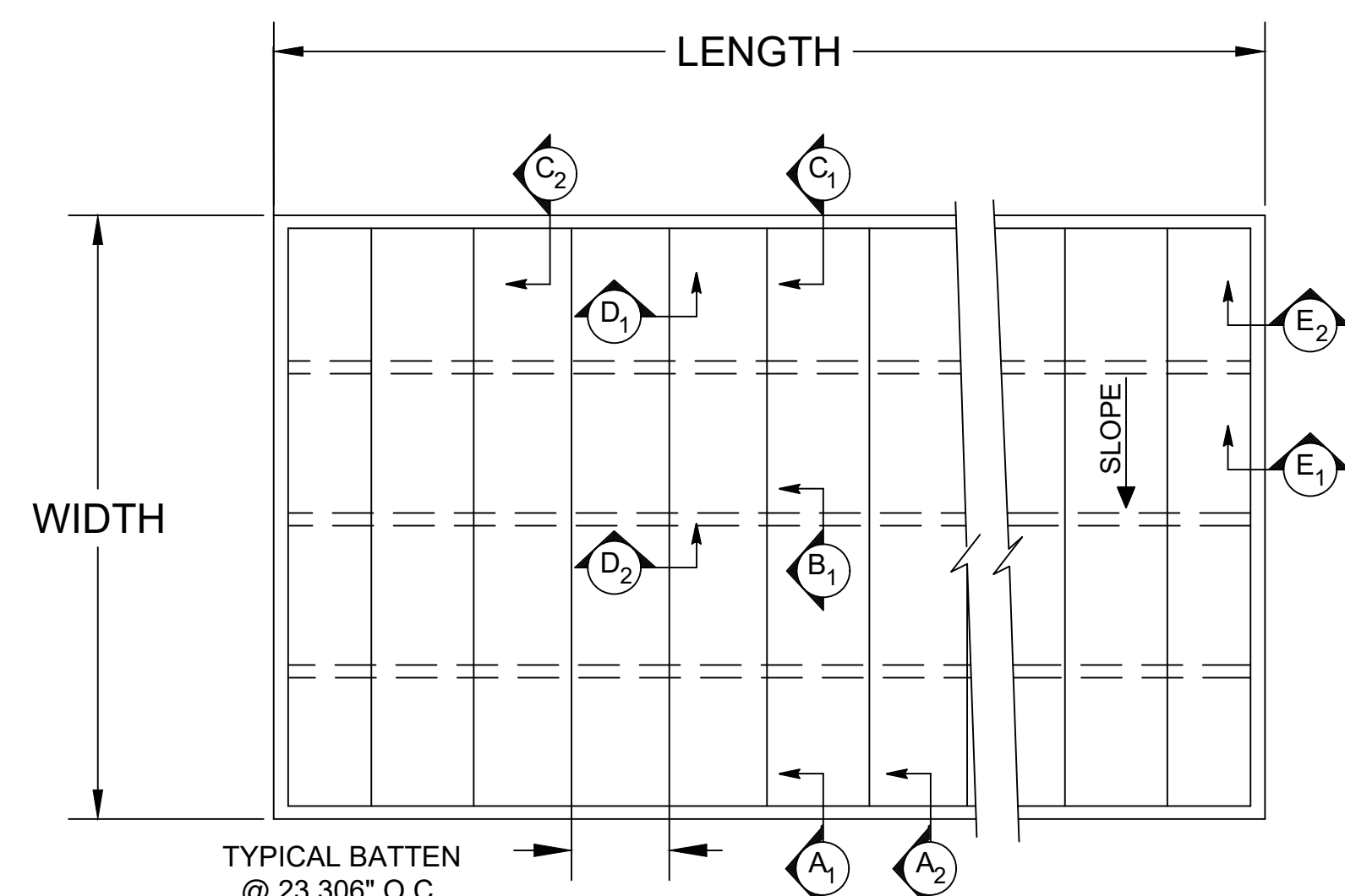
PLANVIEW
