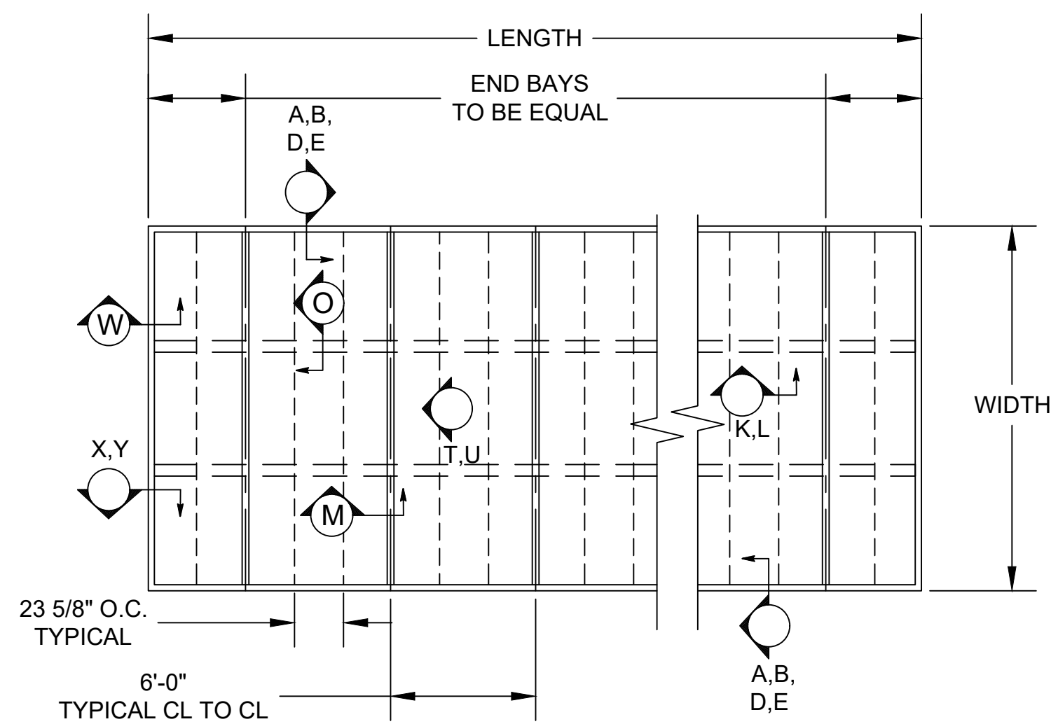
PLANVIEW
