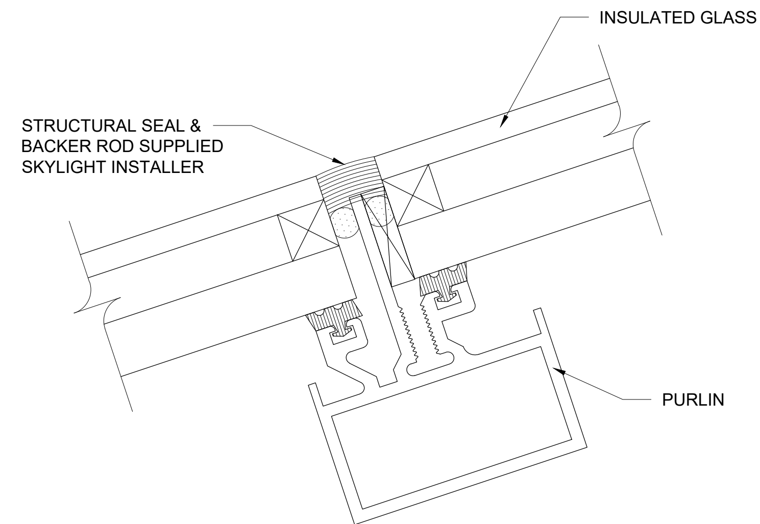
4 1 - - PURLIN DETAIL SCALE: 6" = 1'-0"
