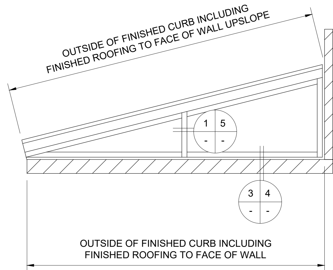
1 1 - - UNIT SECTION SCALE: 6" = 1'-0"
