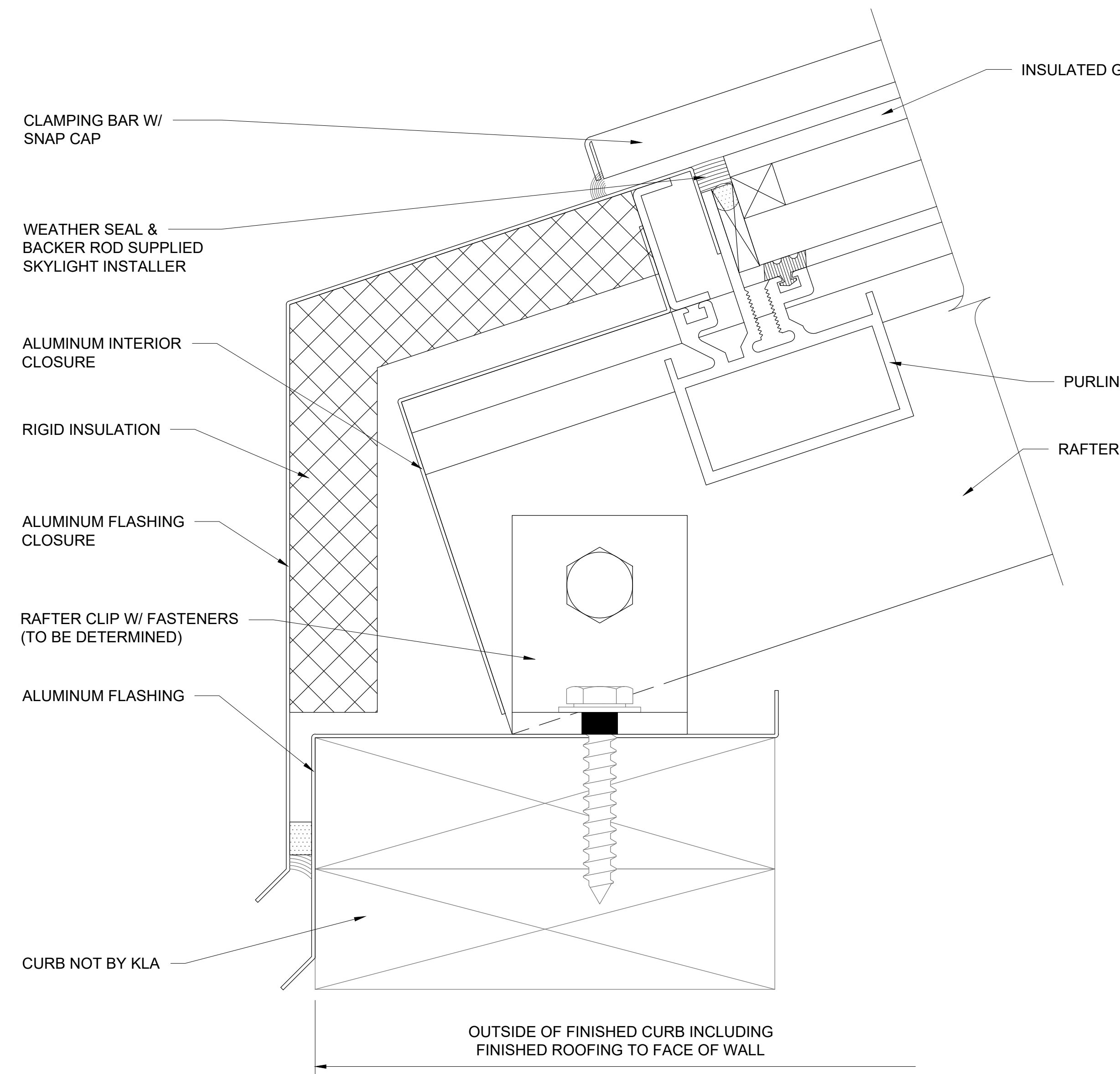
1 2 CURB DETAIL - - SCALE: 6" = 1'-0"
