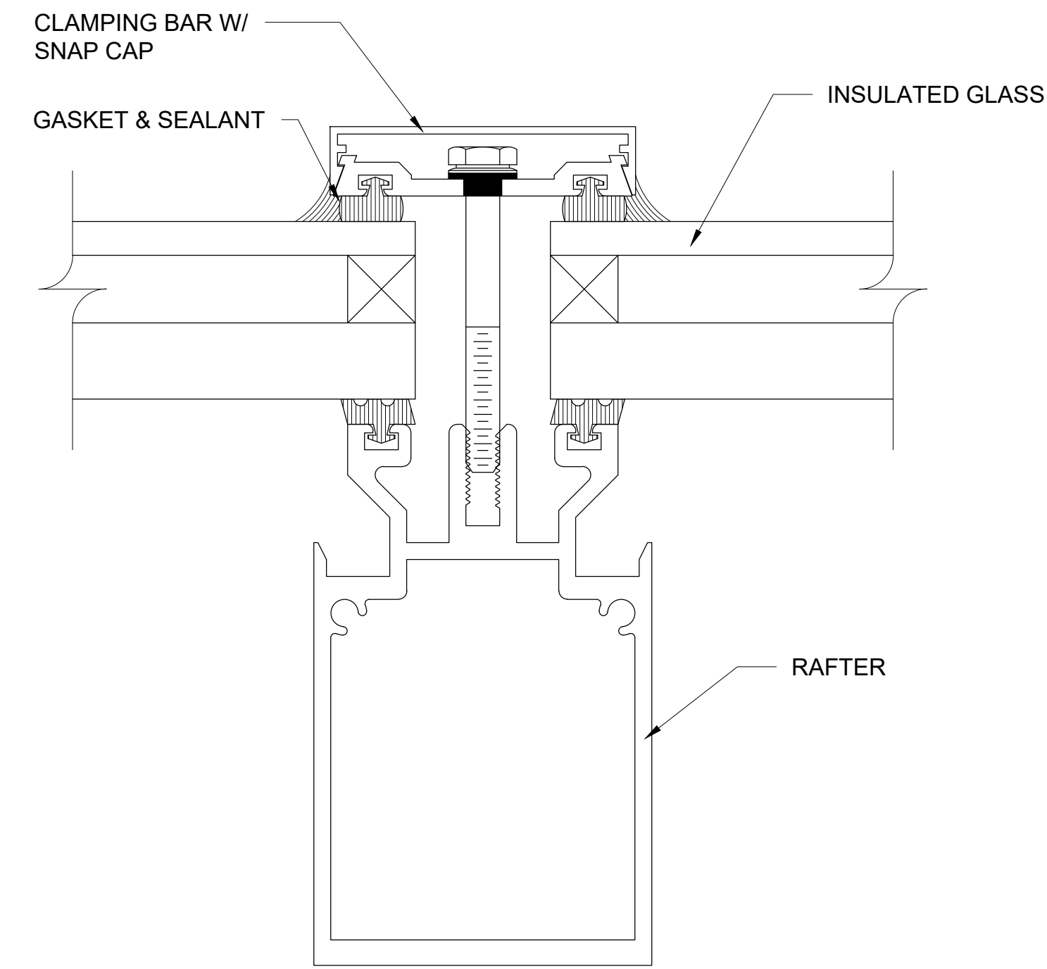
3 1 - - RAFTER DETAIL SCALE: 6" = 1'-0"
