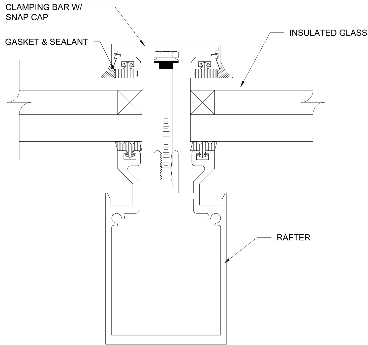
2 2 - - RAFTER DETAIL SCALE: 6" = 1'-0"
