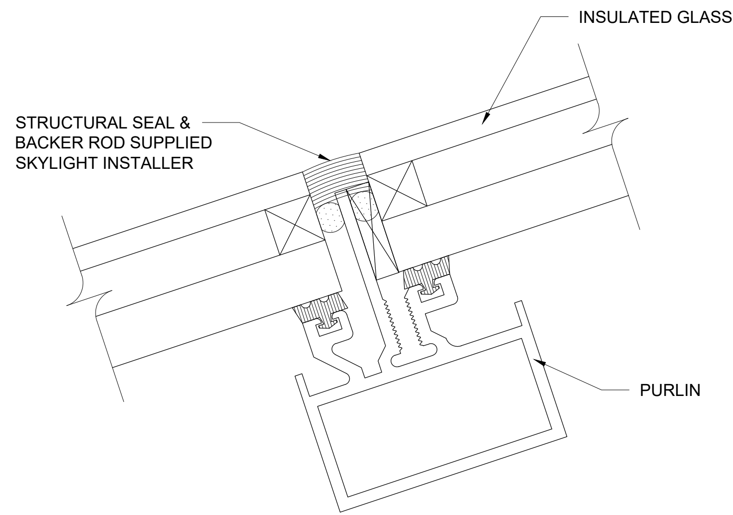
1 2 - - PURLIN DETAIL SCALE: 6" = 1'-0"
