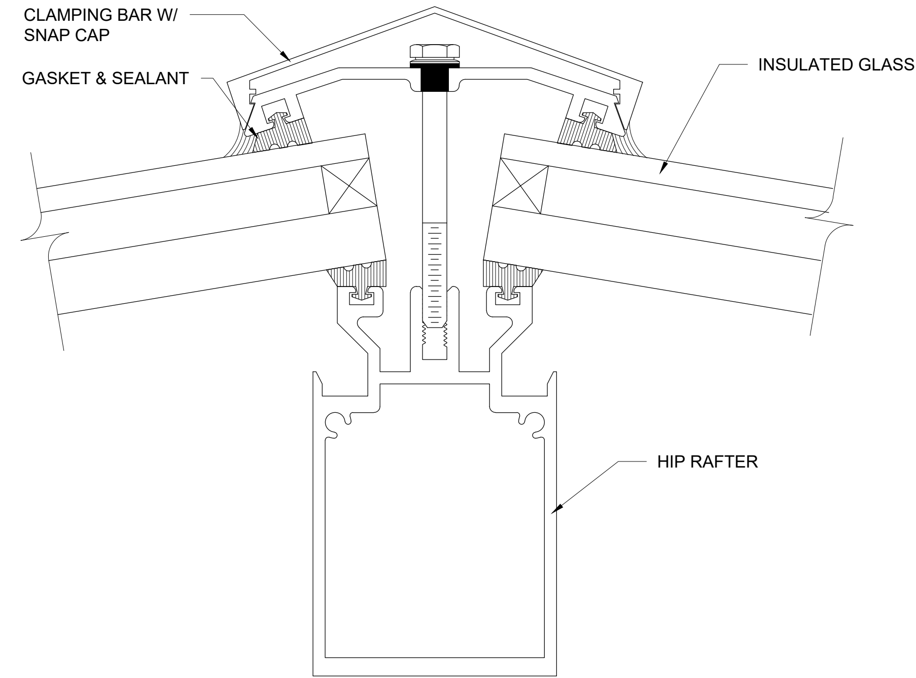
3 2 - - HIP DETAIL SCALE: 6" = 1'-0"
