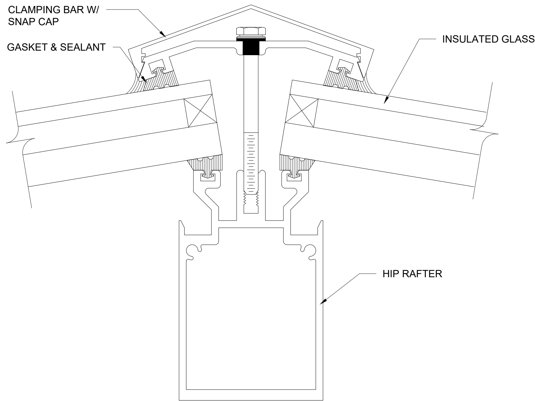
2 2 HIP DETAIL - - SCALE: 6" = 1'-0"
