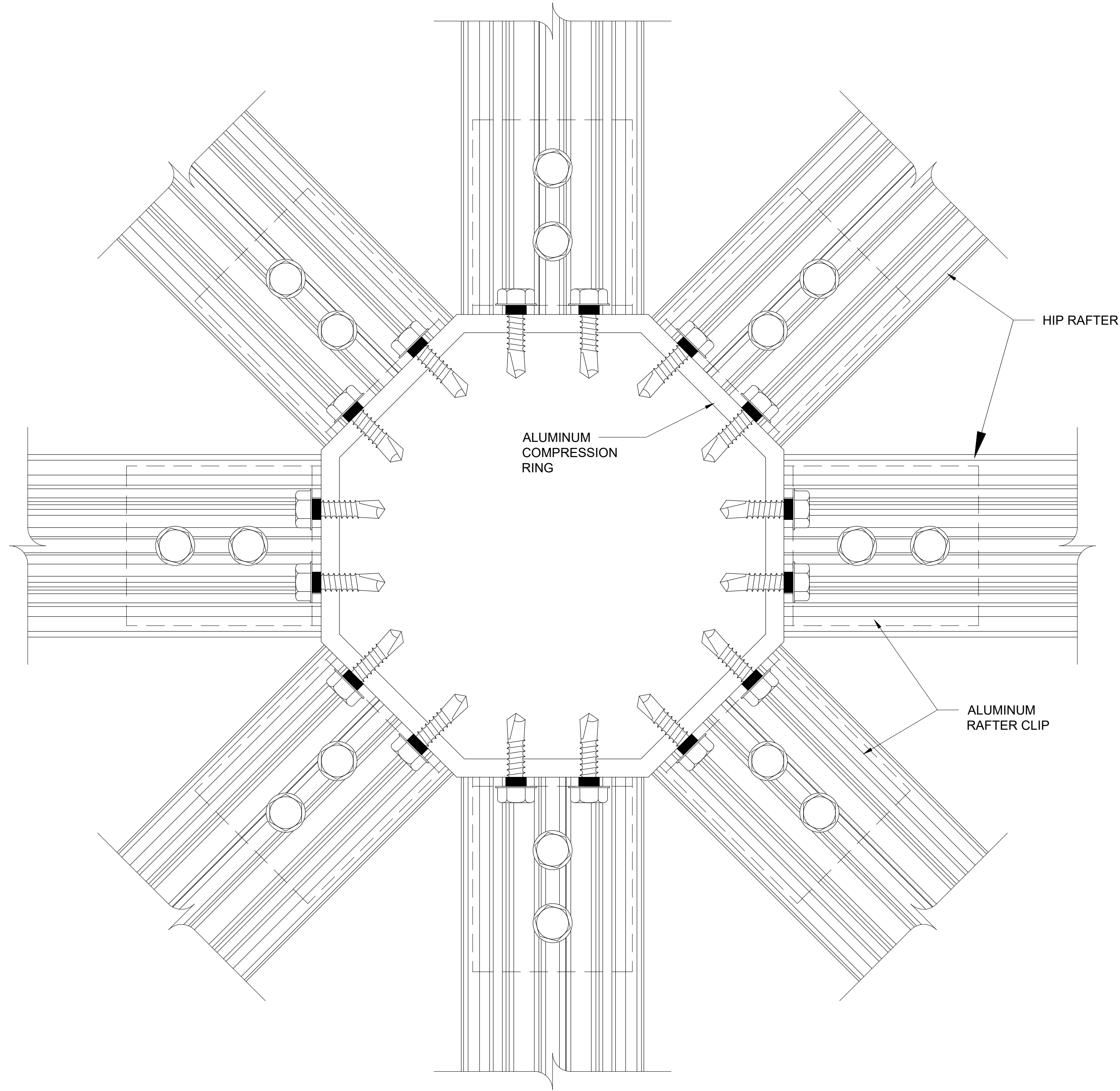
1 3 COMPRESSION RING - - SCALE: 6" = 1'-0"
