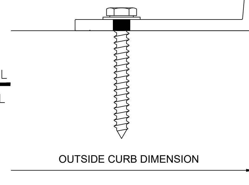
4 2 - - CURB DETAIL SCALE: FULL
