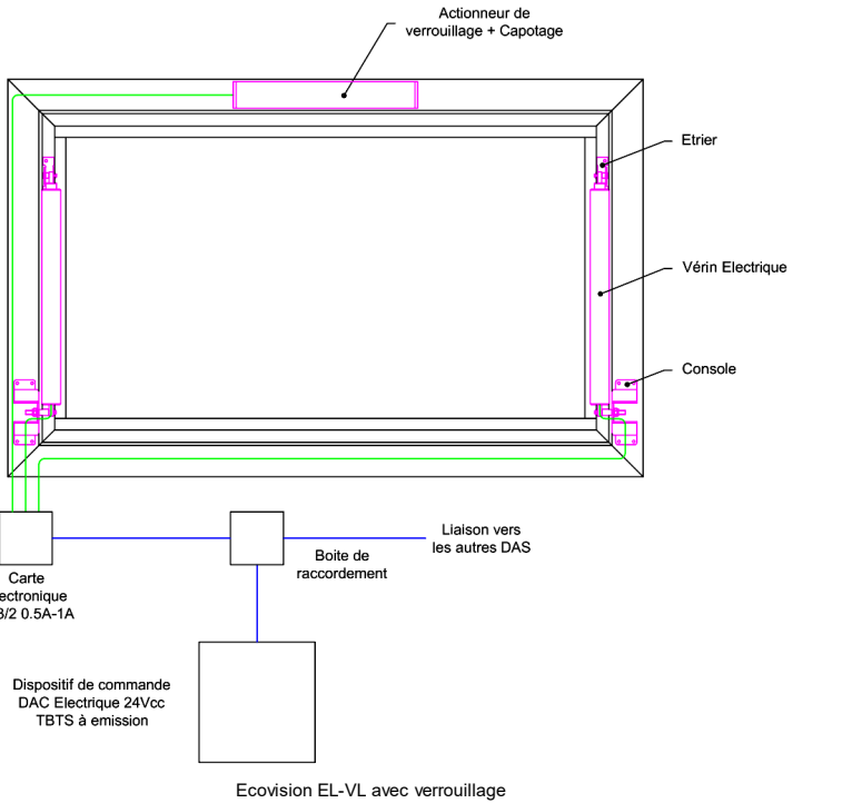
Ecovision EL-VL avec verrouillage
